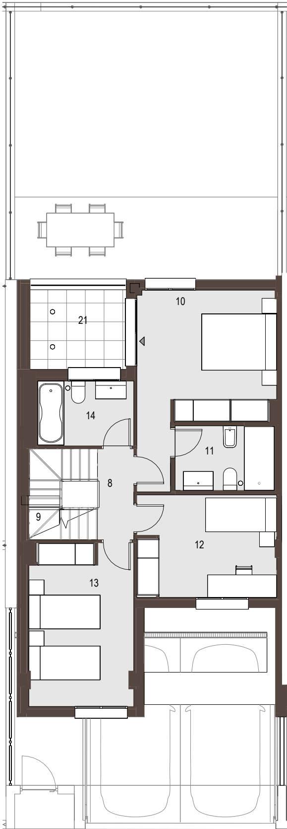
P01 - PLANTA PRIMERA
